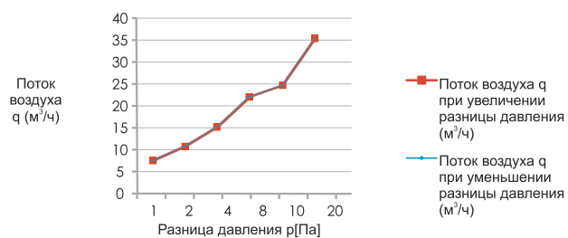
График 10. Зависимость потока воздуха q ( \text{м}^3/\text{ч} ), протекающего через клапан VT 1001, от разницы давления p (Па)
