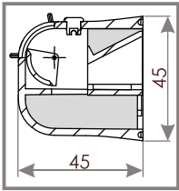
PRZEKRÓJ VT 400
