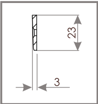
PRZEKRÓJ OZ 300
