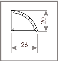
PRZEKRÓJ OZ 100
