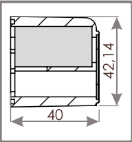
PRZEKÓJ OZ 400
