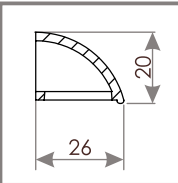
PRZEKRÓJ OZ 300
