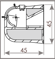
PRZEKÓJ LA 100
