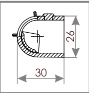
PRZEKRÓJ OZ 200
